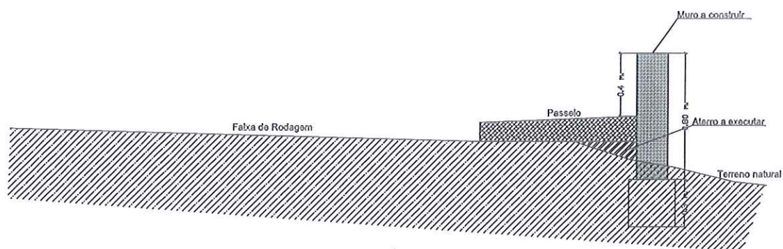
Corte - S/Esc
