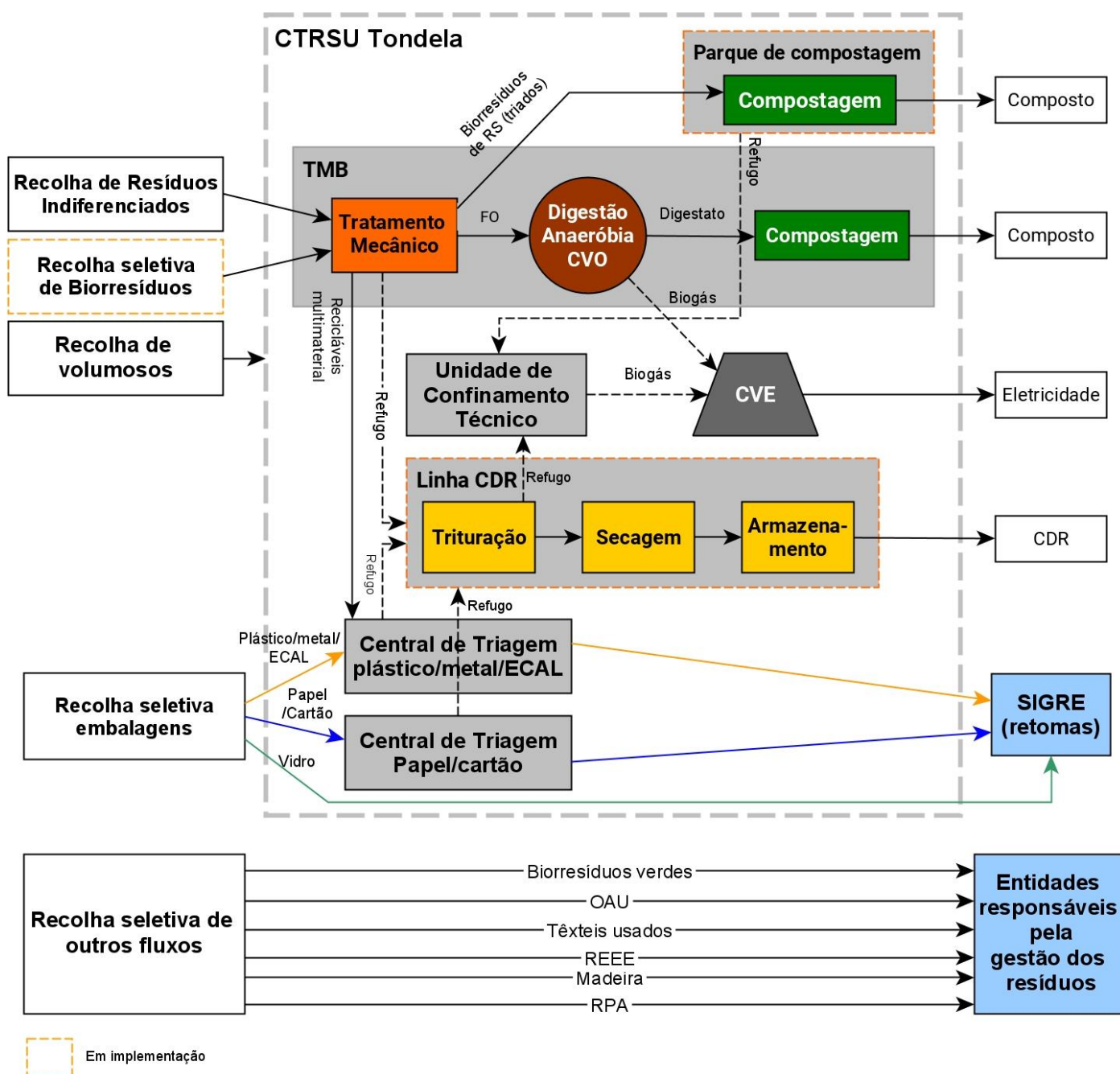
Figura 10 – Esquema ilustrativo do funcionamento do modelo técnico de gestão de RU no território da EG.
